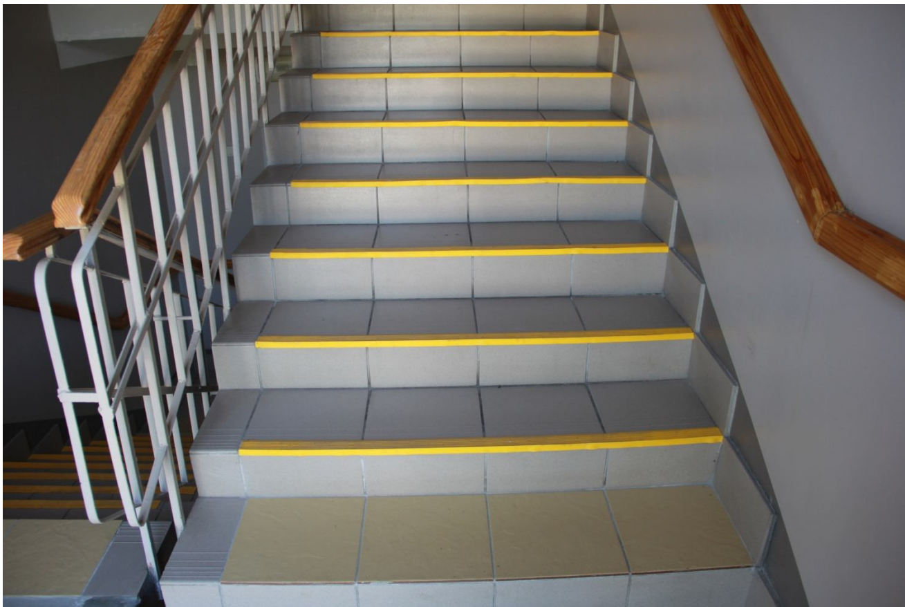
Лестничные марши с выделением цветом краевых ступеней, краёв ступеней
